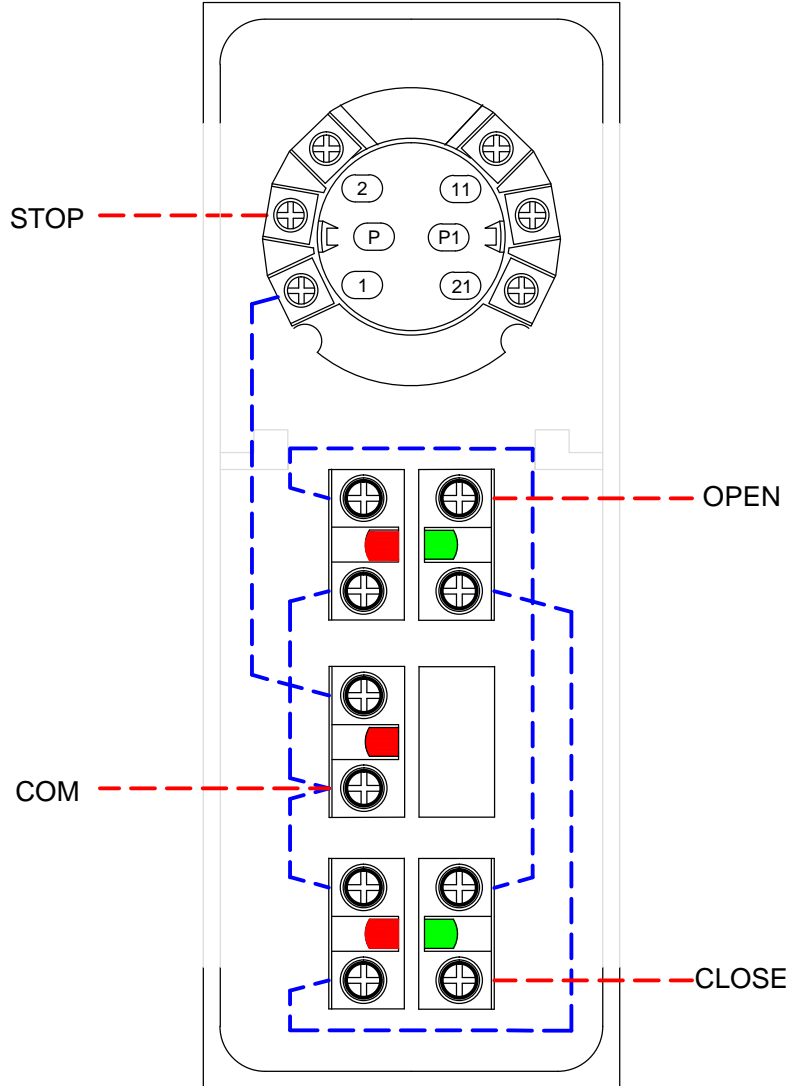
N.O Switch
